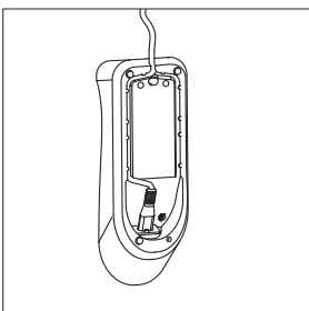
Obrázek 4: Připojení síťového kabelu (na spodní straně nabíjecí stanice)
