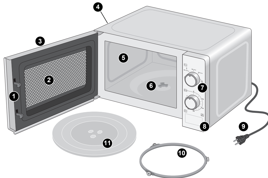
Abb. 1: Elementy urządzenia
