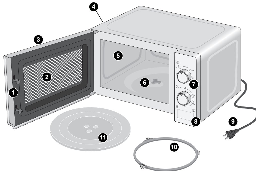
Abb. 1: Компоненты прибора
