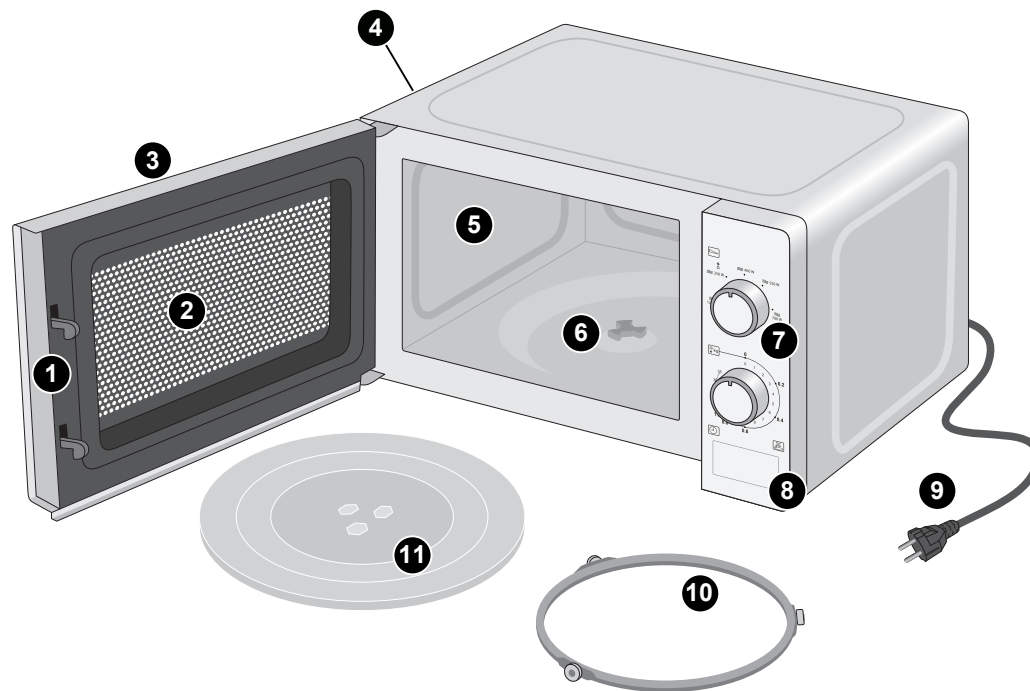
Abb. 1: Parti dell'apparecchio
